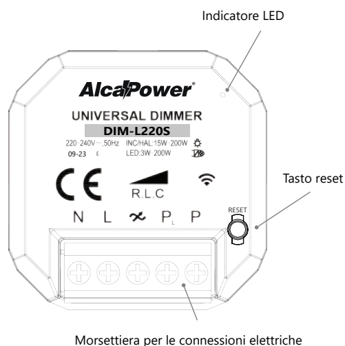
Morsetteria per le connessioni elettriche
